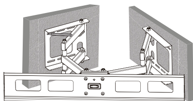
Fig. 1: Ausrichten und Anzeichnen
