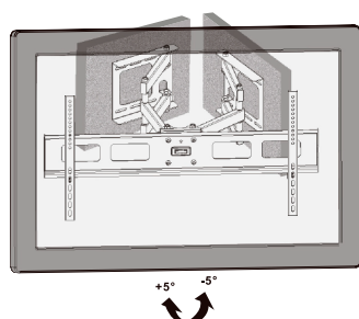
Fig.40: Allineare e fissare dello schermo piatto
