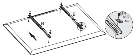
Fig. 25: Ecrans plats avec face arrière plane 2
