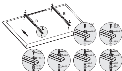
Fig. 7: Flachbildschirme mit gewölbter Rückseite 2
