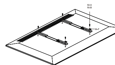
Fig.5: Flachbildschirme mit flacher Rückseite 2
