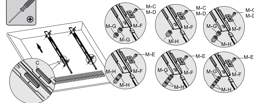
Fig. 15: Schermi piatti con fondo curvo
