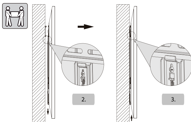
Fig. 4: Einhängen des Flachbildschirms
