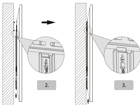
Fig. 16: Fissare dello schermo piatto
