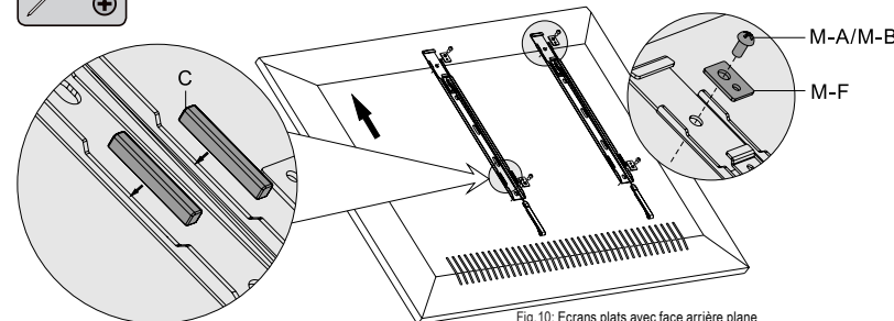
Fig.10: Ecrans plats avec face arrière plane
