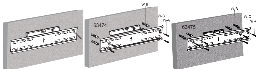
Fig. 13: Installazione su parete
