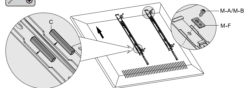
Fig. 2: Flachbildschirme mit flacher Rückseite
