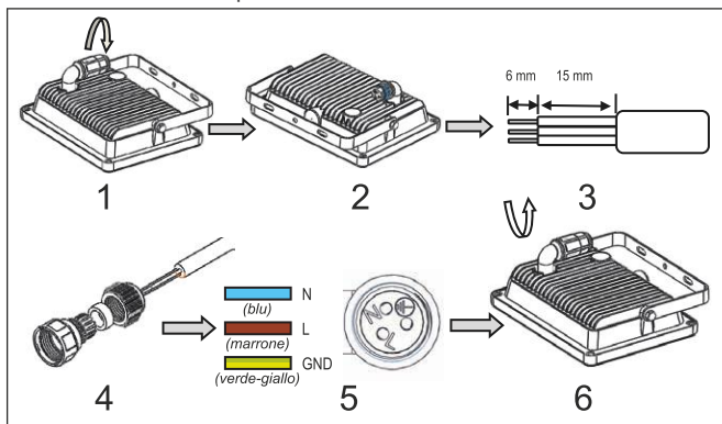
Fig.28: Installazione fissa
