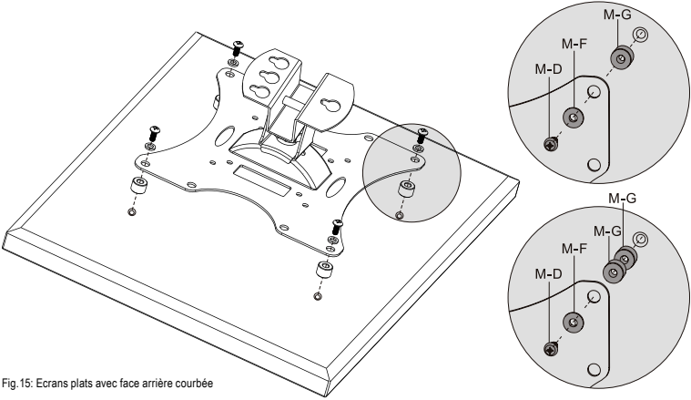
Fig.15: Ecrans plats avec face arrière courbée
