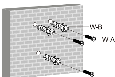
Fig. 18: Installazione su parete
