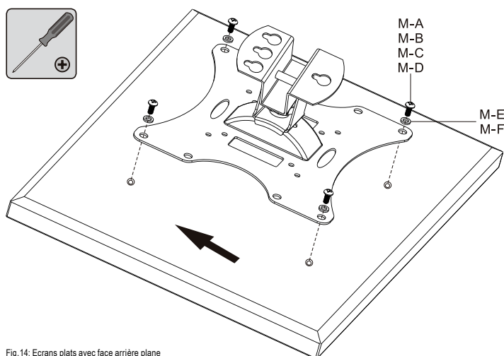
Fig. 14: Ecrans plats avec face arrière plane
