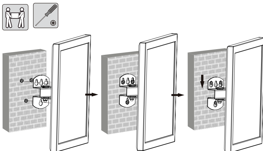
Fig. 5: Einhängen und Sichern des Flachbildschirms
