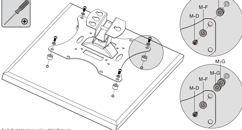
Fig.3: Flachbildschirme mit gewölbter Rückseite
