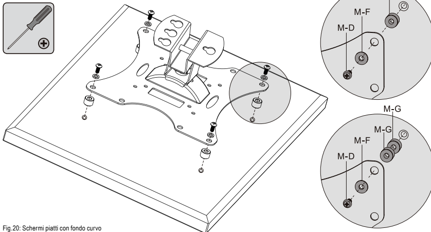
Fig.20: Schermi piatti con fondo curvo
