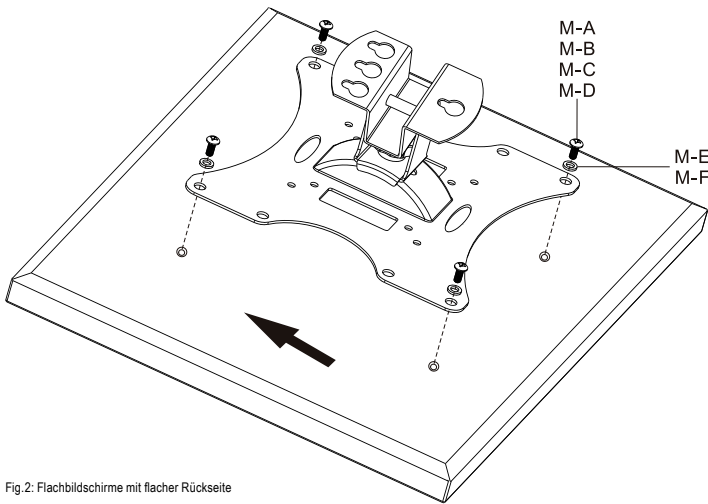
Fig.2: Flachbildschirme mit flacher Rückseite
