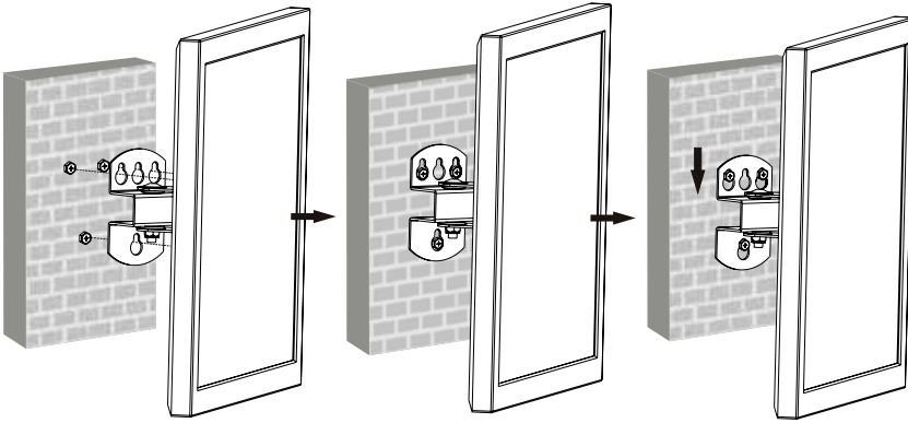
Fig. 16: Assembler et fixer l'écran plat
